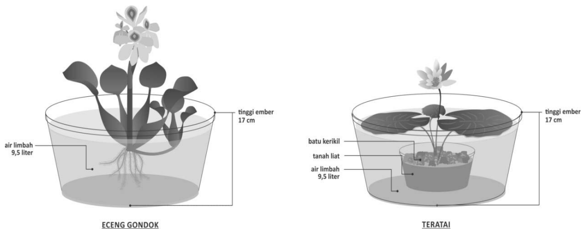
Gambar 1. Simulasi penelitian
