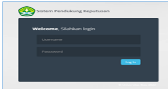
Gambar 2 Tampilan Login
