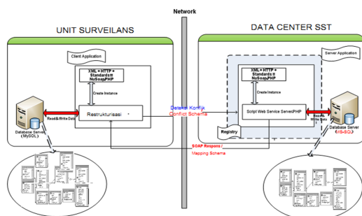
Gambar 6. Deteksi Konflik Skema level instance
