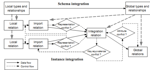
Gambar 3. Proses Integrasi Skema
