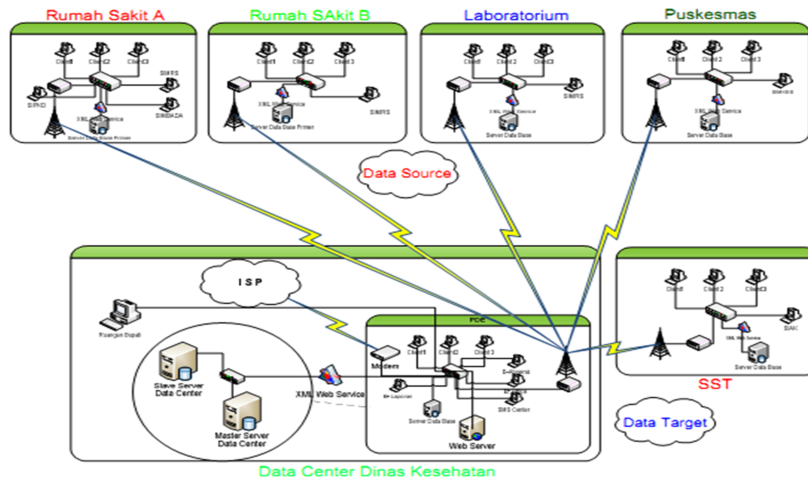
Gambar 5. Arsitektur Integrasi Epidemiologi
