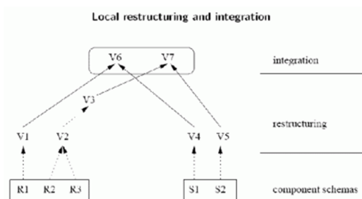
Gambar 1. Bagan Proses Restrukturisasi dan Integrasi Basis Data
