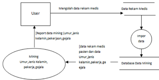
Gambar 2. DFD level 1
