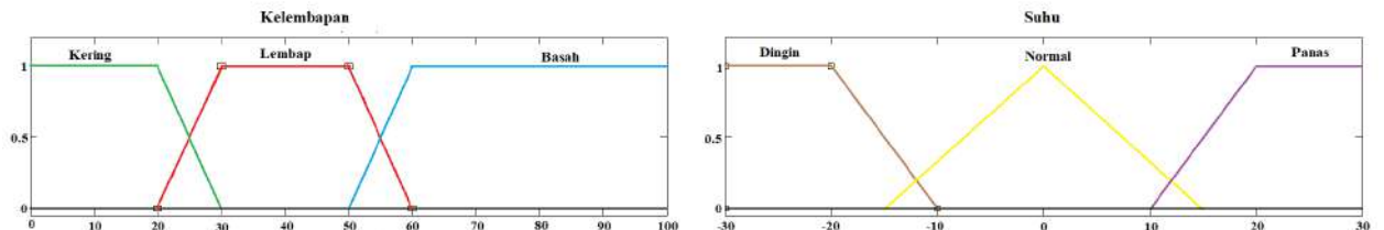
Gambar 8 Fungsi Keanggotaan Input suhu dan kelembapan
