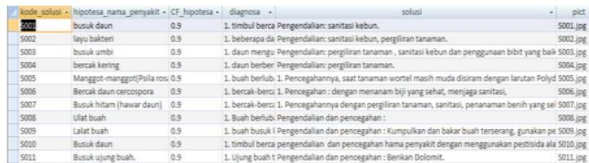
Gambar 6 : table solusi
