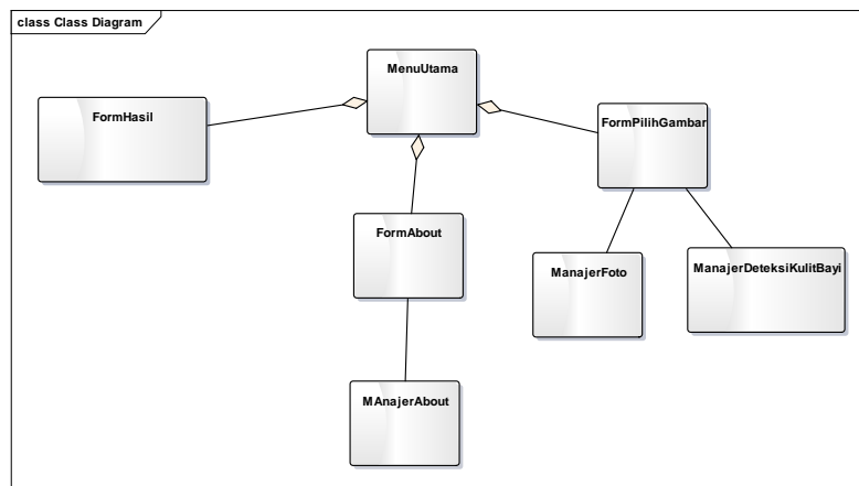
Gambar 6 Class Diagram Aplikasi
